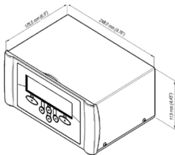
Монохромный контроллер
